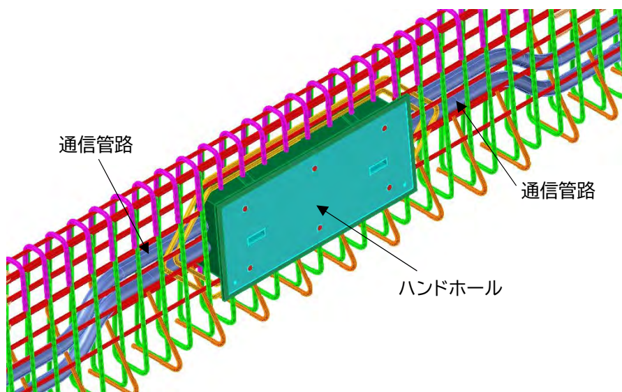
図-3.8.1 ハンドホールの設置概念図
