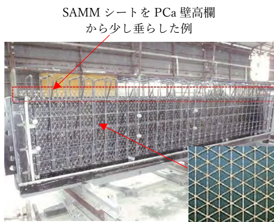
写真-4.4.1 SAMM シートの配置例
