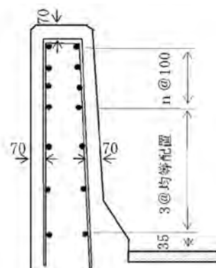
図-3.6.10 横方向鉄筋の配置図
