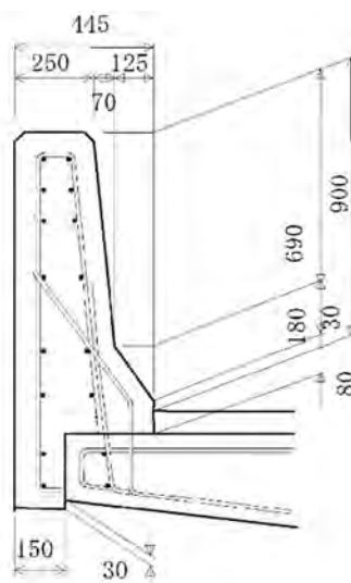
(b) PC床版の場合
