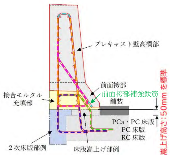
図-7.2.1 標準化の断面形状
