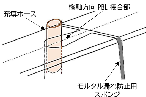
図-1.2.3 充填ホースの差し込み口
