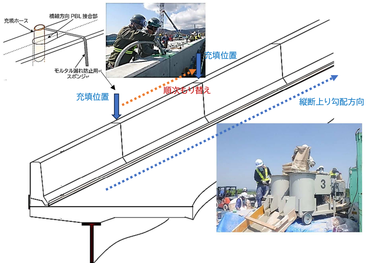
図-2.5.1 充填ホースのもち替え例
