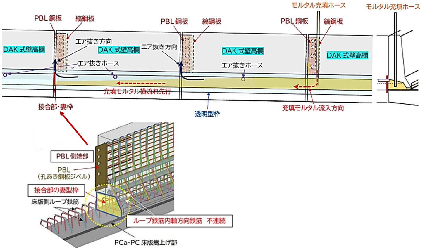
図-2.5.11 橋軸方向の横流れ先行を抑制するための妻型枠設置例
