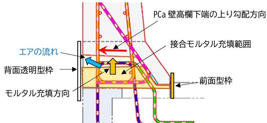
図-1.2.1 前面袴を有する場合の標準的な型枠設置図
