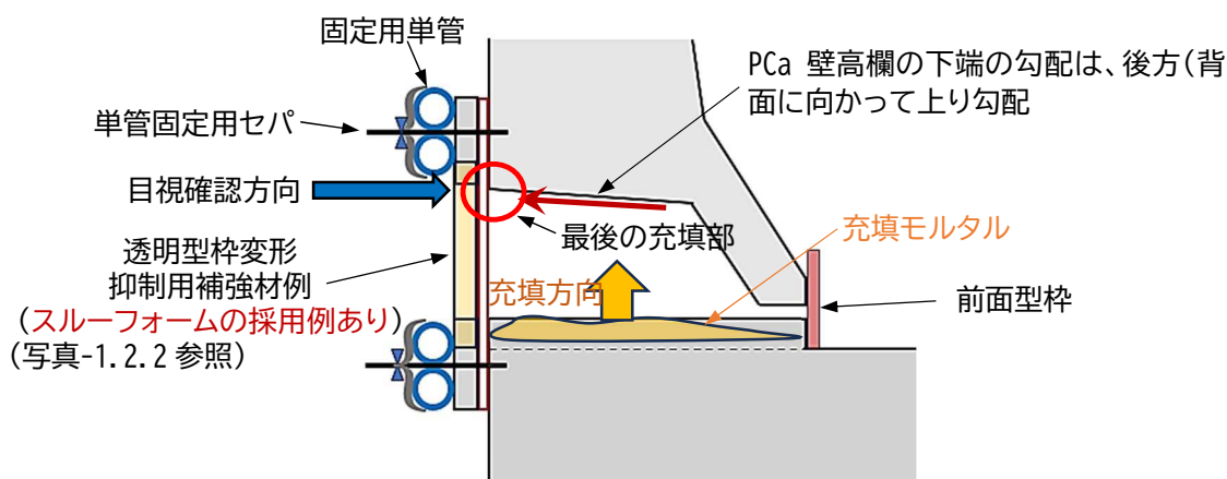
図-1.2.2 前面枠を有する場合の透明型枠設置と型枠固定の例
