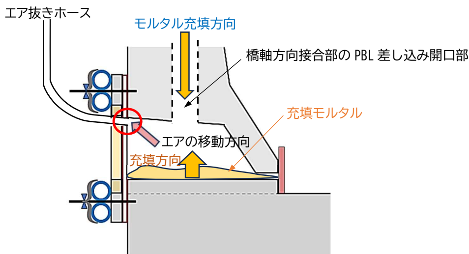
図-1.2.4 前面袴を有する場合の透明型枠のエア抜き対策
