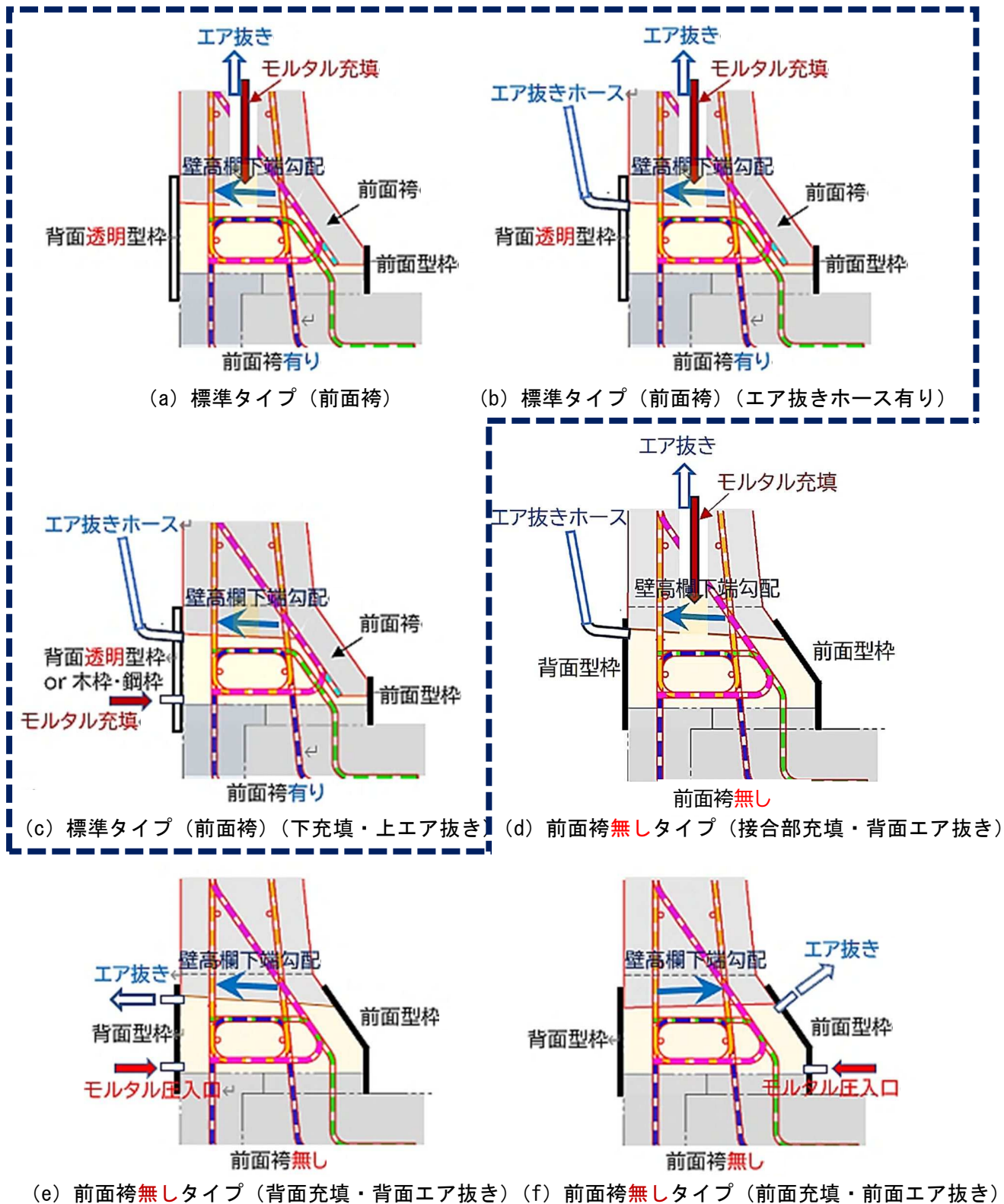
図-2.5.2 床版接合部のモルタル充填方法の実績
