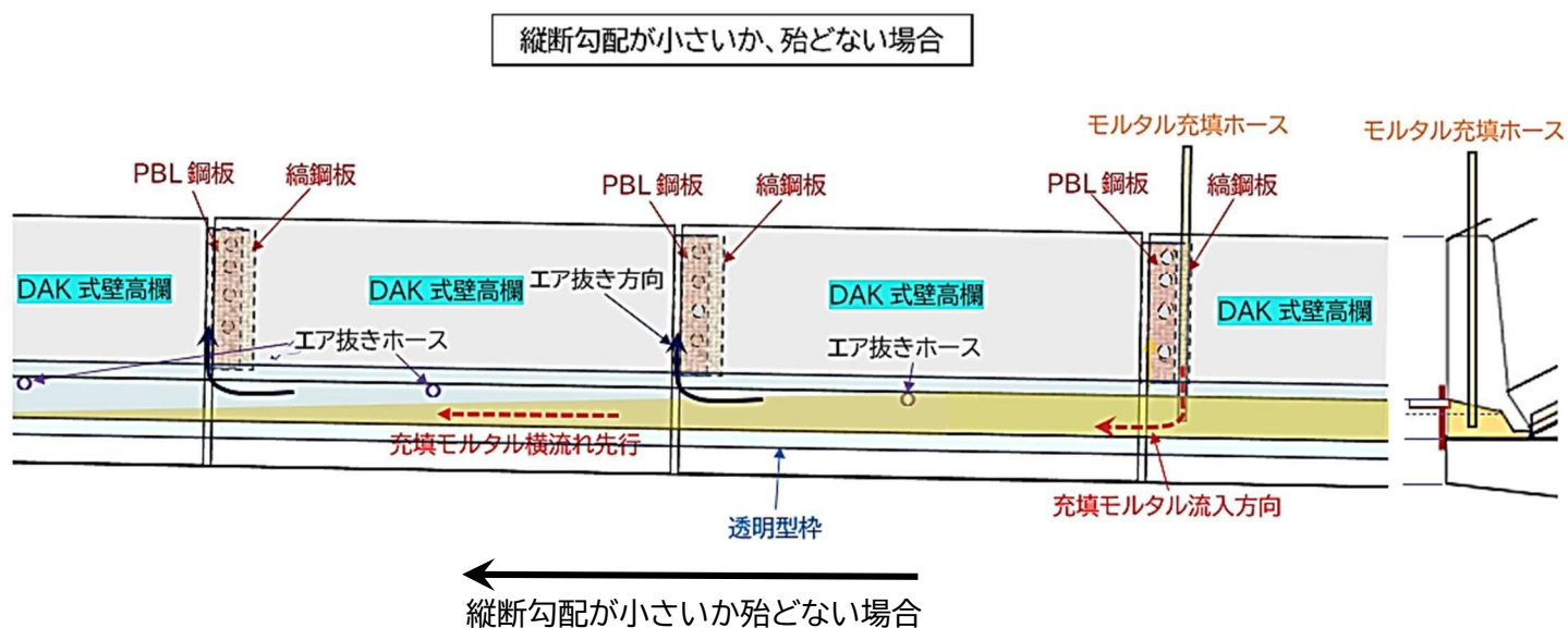
図-2.5.10 橋軸方向横流れが先行するモルタル充填状況図例
