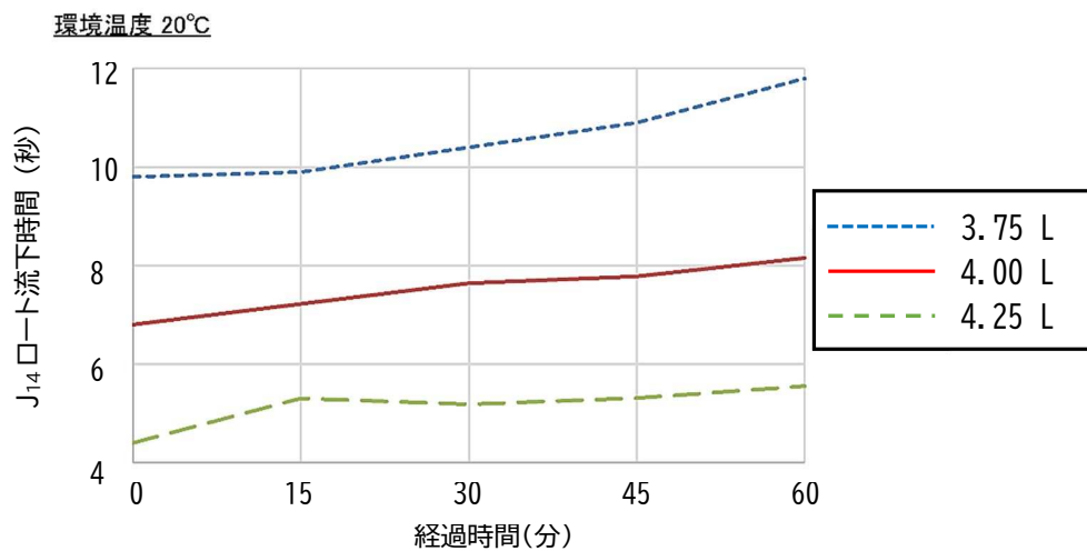
図-2.4.1 J 14 ロートにおける流下時間の経時変化の計測例
